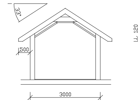
SNITT ARK
