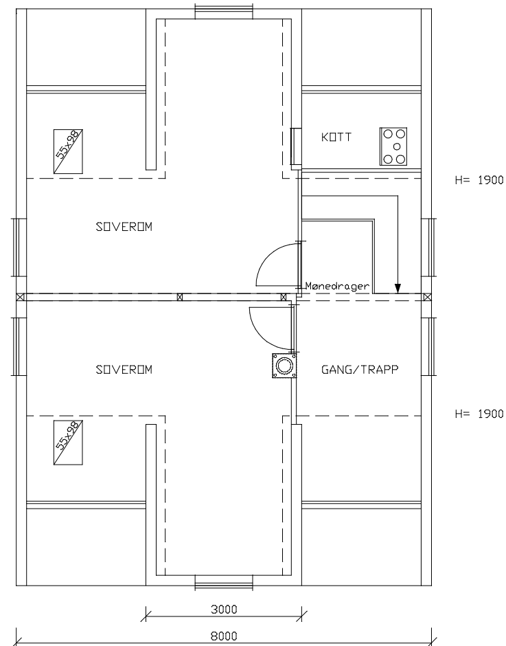
LOFTSPLAN
