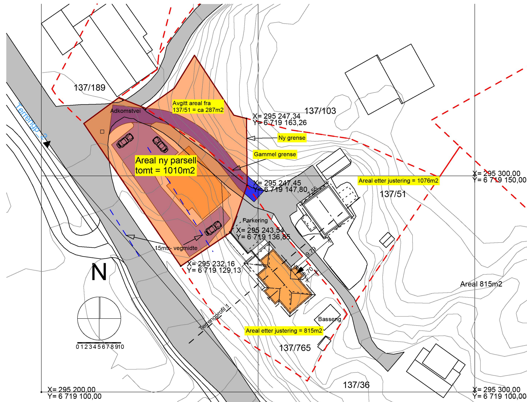
Situasjonsskisse, 1:500
