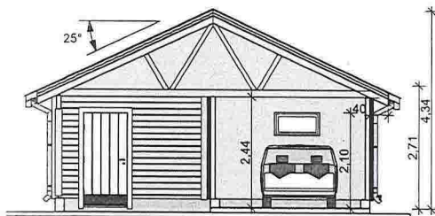
Snitt A-A
