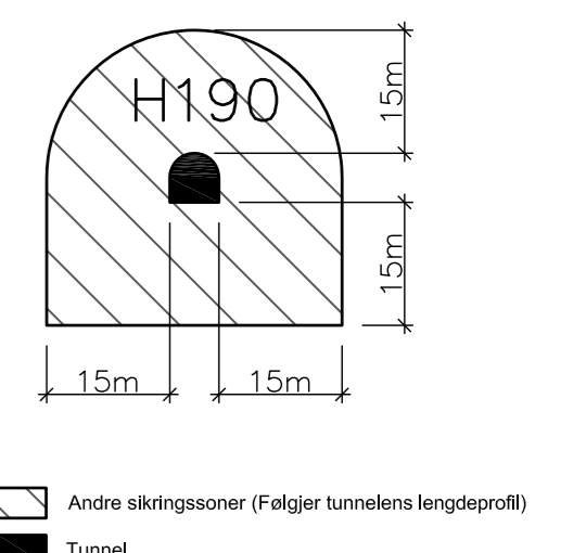
PRINSIPPSNITT FOR ANDRE SIKRINGSSONER (H190) M=1:1000
