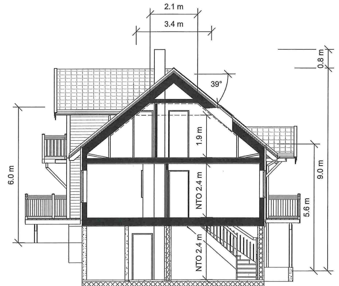
SNITT A-A
