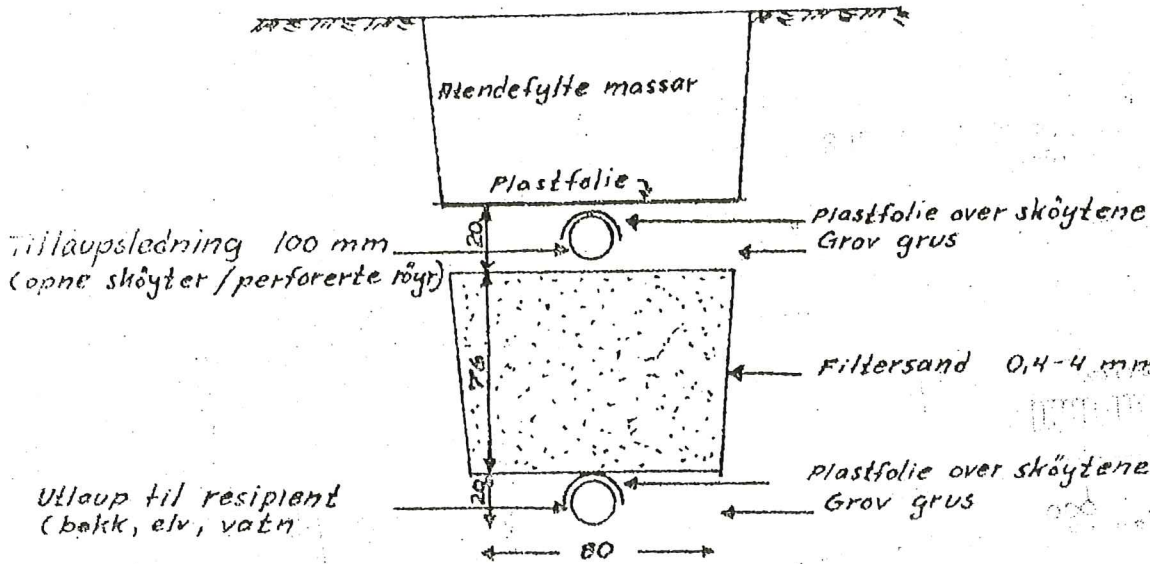
Fig. 7. Sandfiltergrøft (Alle mål i cm) Maks fall 1 cm på 5 m
