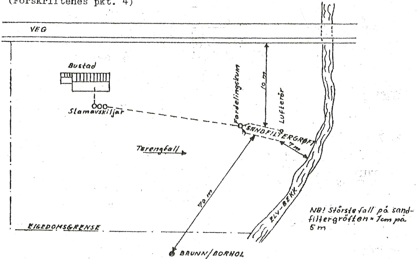
Fig. 5. Prinsippiel skisse av systemet. (Alle mål er minimumsavstander)
