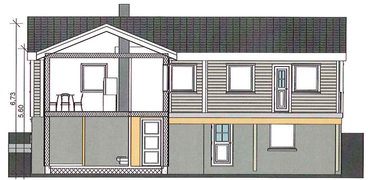
Snitt BB
