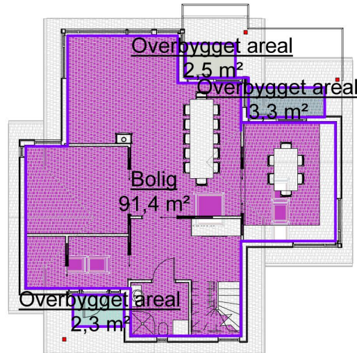
3 Plan 1 - BRA 1 : 200
