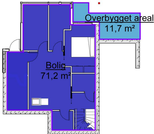
2 Plan 0 - BRA 1 : 200
