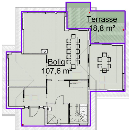
1 BYA 1 : 200
