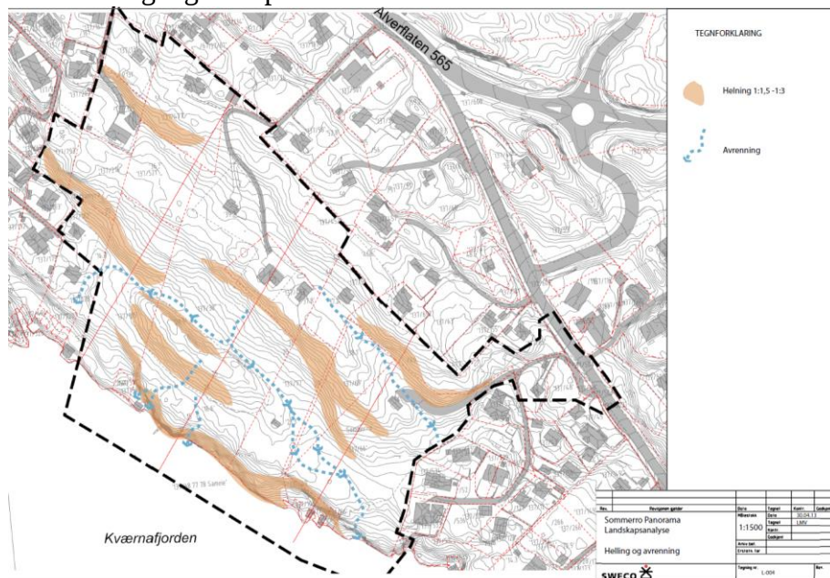
Bilde: Hellingkart som viser helning 1:1,5 og 1:3 og avrenning. Kjelde Sweco
