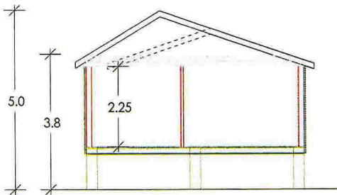
Snitt A-A
