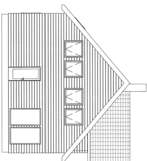
Fasade Nord 1 : 100
