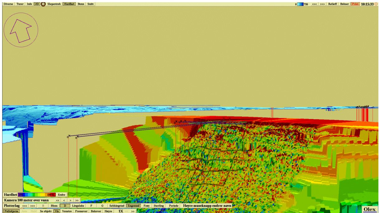
Figur 6. 3D skisse bunntopografi under anlegg med hardhet.
