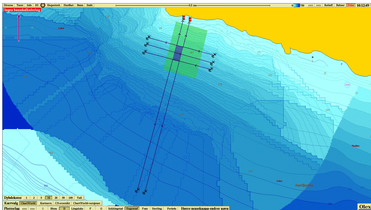
Figur 4. Undervannstopografi ved lokaliteten. Lakseanlegget med flytekrager med en omkrets på 160m er inntegnet på lokalitet.
