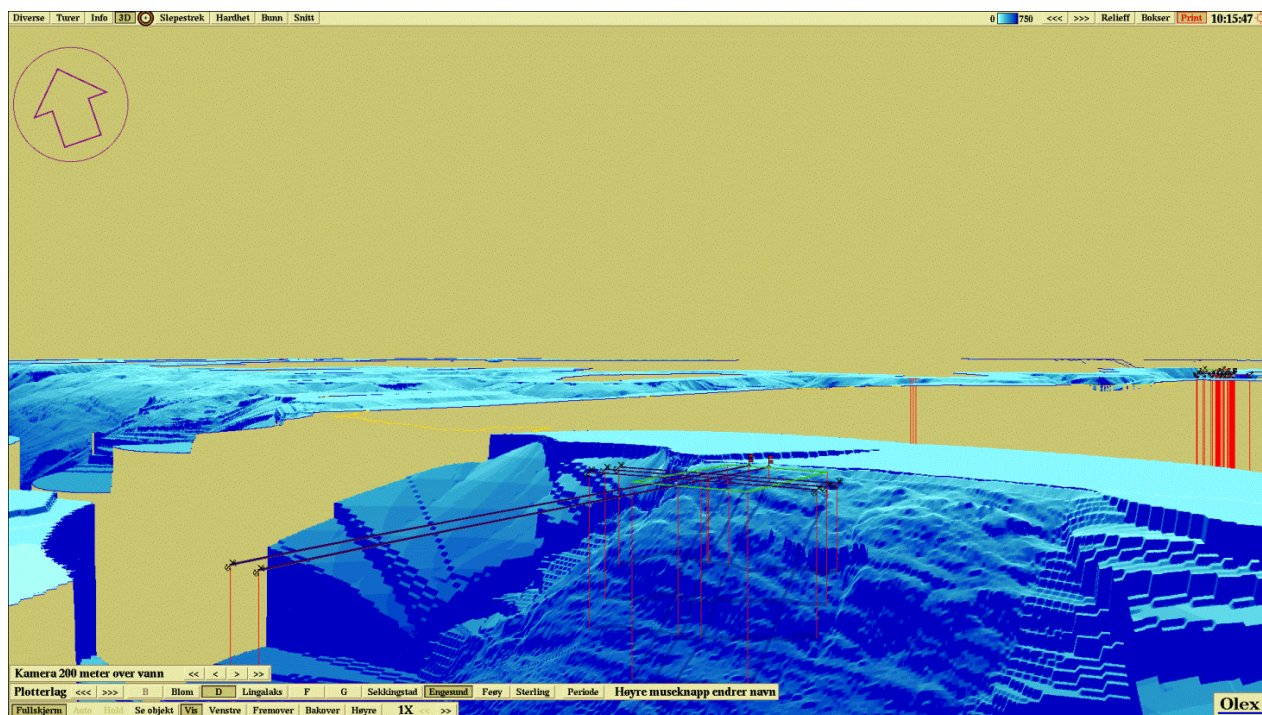
Figur 5. 3D skisse med bunntopografi under lakseanlegget med fortøyningslinjer.
