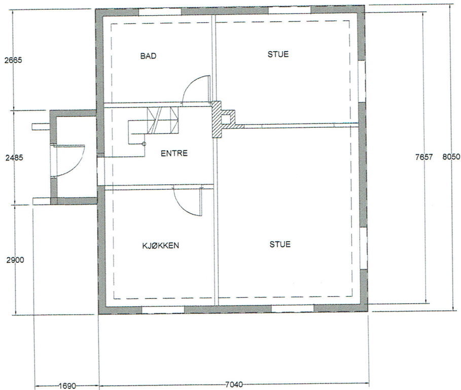
EKSISTERENDE HOVEDPLAN
