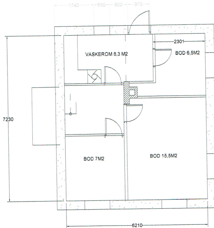
EKSISTERENDE KJELLERPLAN
