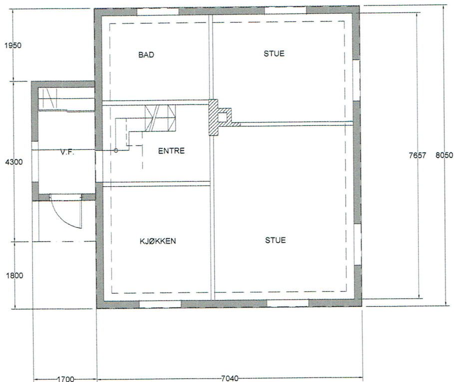
NYTT HOVEDPLAN
