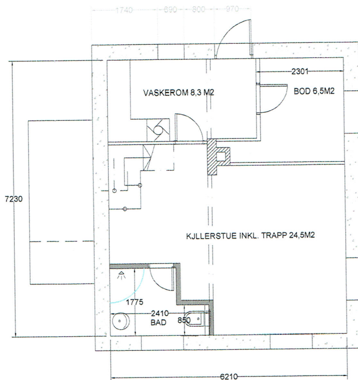
NY KJELLERPLAN
