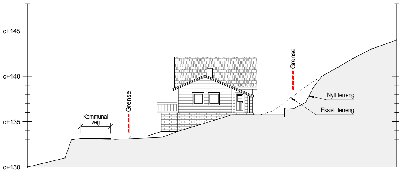
PROFIL A
