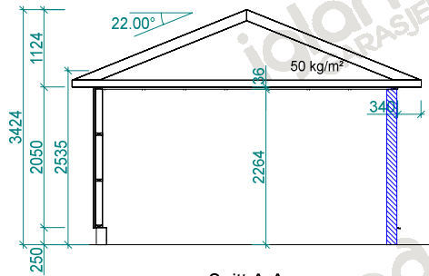
Snitt A-A
