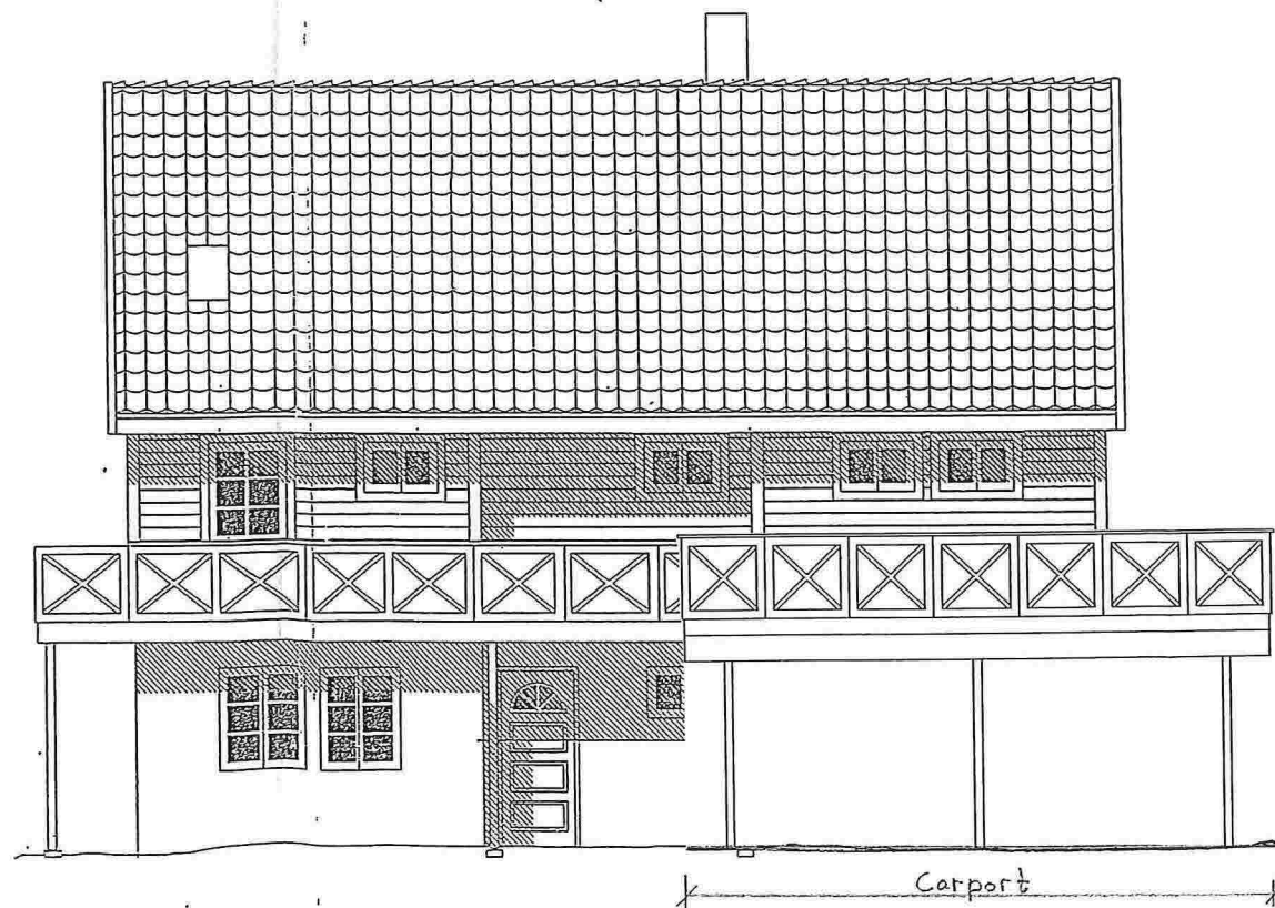
FASADE SØR-VEST
