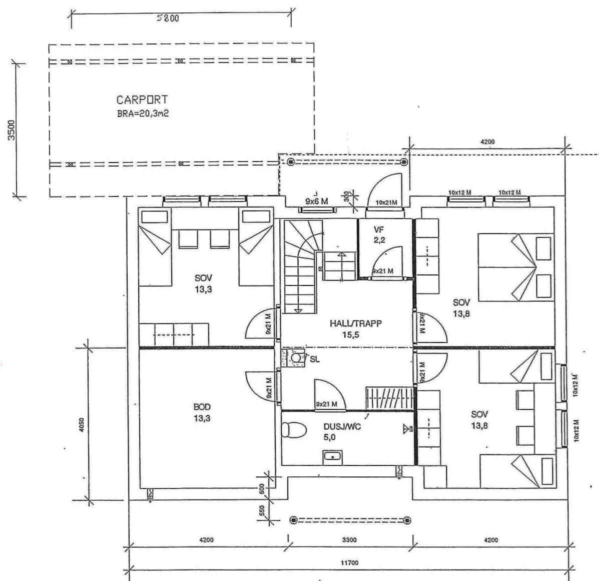
PLAN U.ETG.
