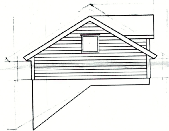
Fasade mot vest
