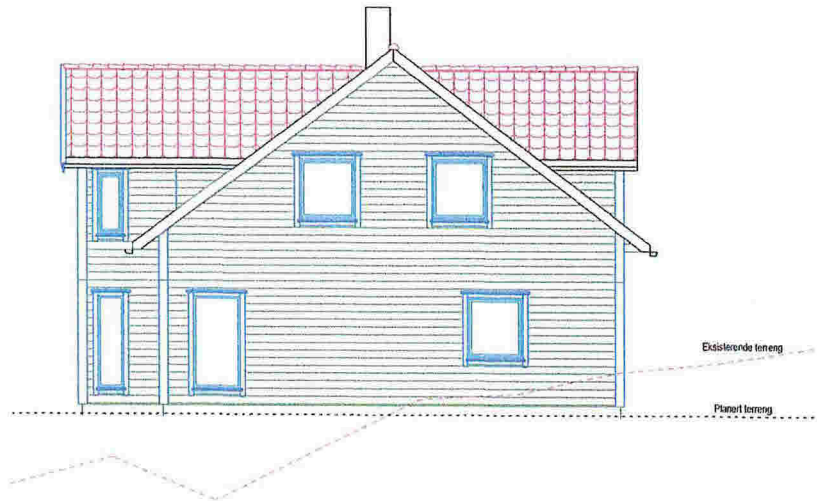
FASADE: ØST
