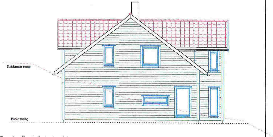
FASADE: VEST
