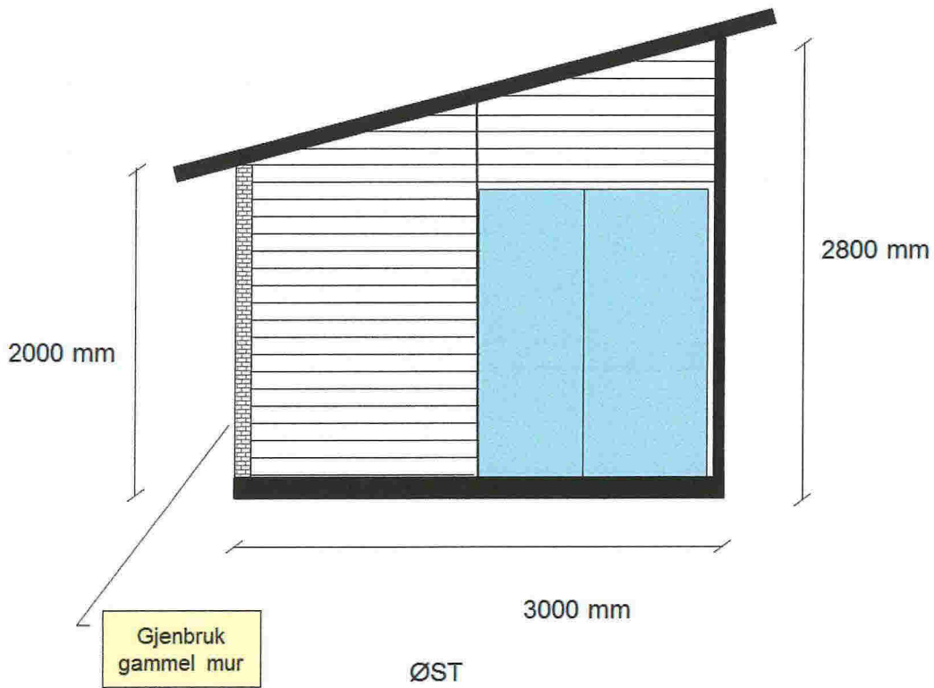
Tegning 3 - Sett fra eksisterende uteplass/bod
