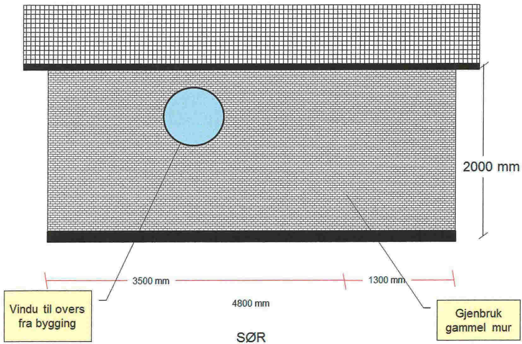
Tegning 4 - Sett fra sør/sørvest (mot 52/59)
