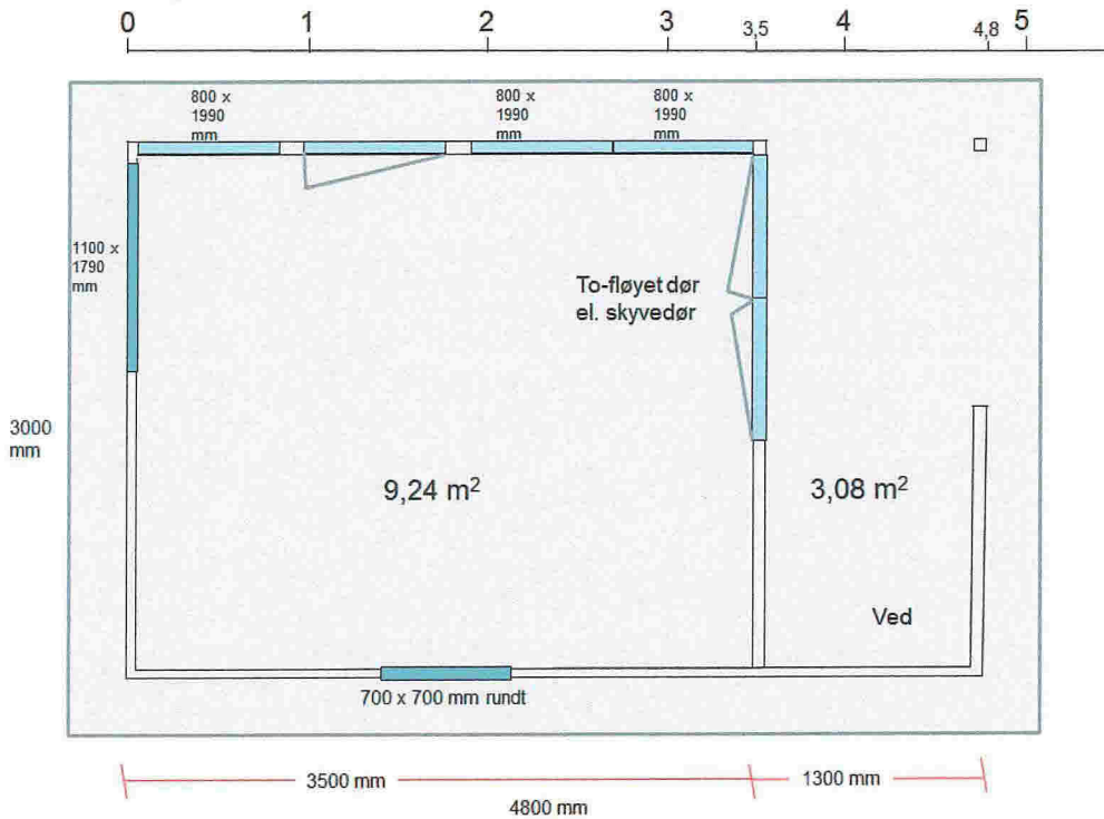
Tegning 1 - Plantegning med mål
