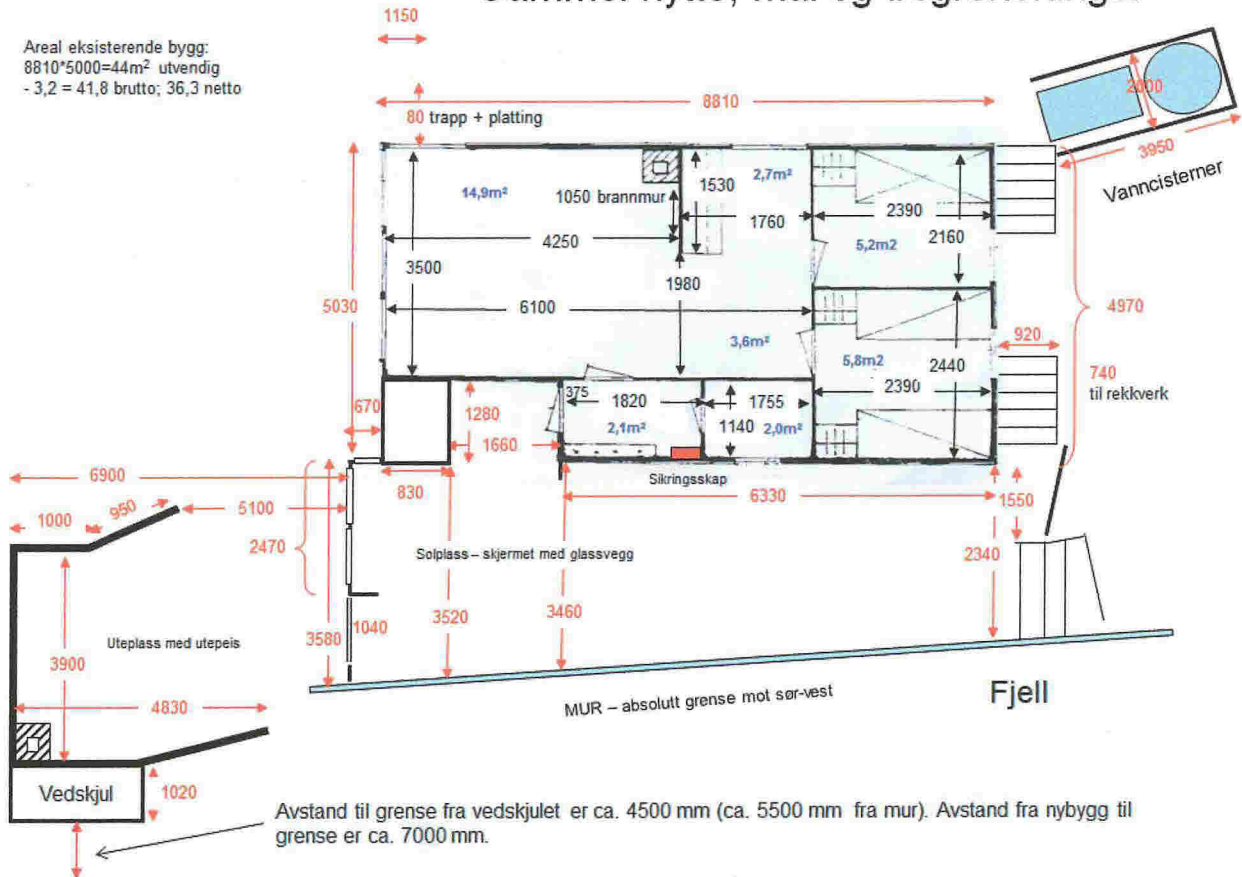
Tegning 1 - Mål på eksisterende mur
