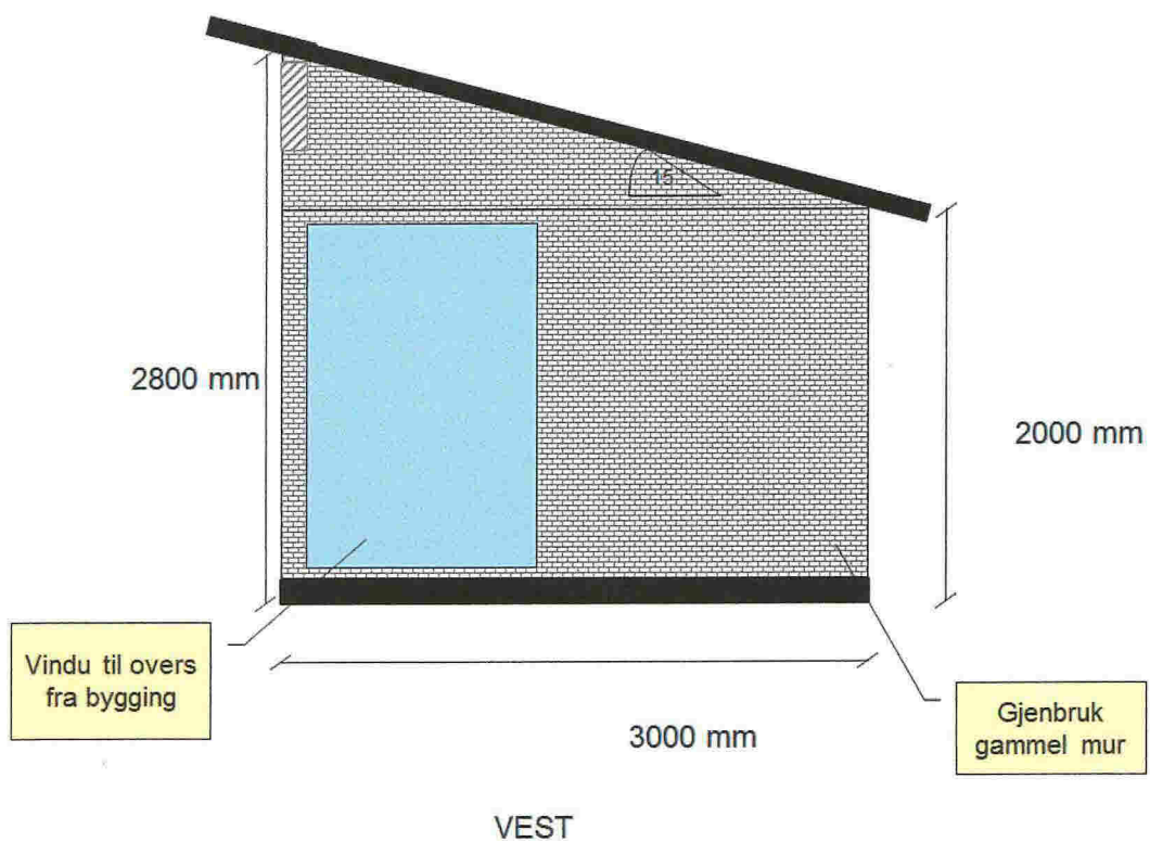
Tegning 2 - Sett fra sjøsiden
