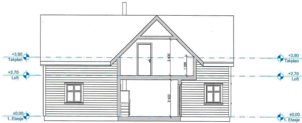
SNITT A-A
