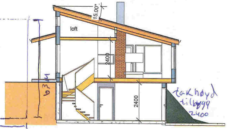
Section 3 1 : 100
