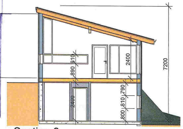
Section 3 1 : 100
