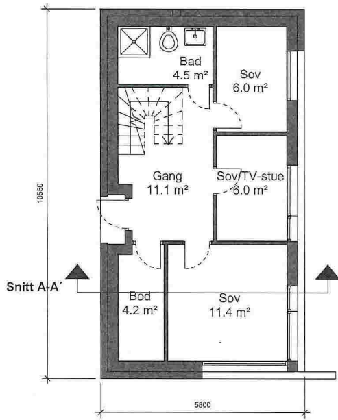
Plan 1. etasje
