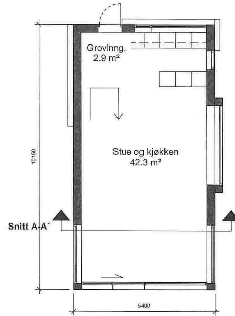
Plan 2. etasje
