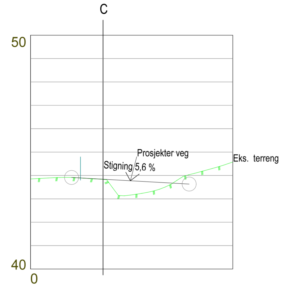
Lengdeprofil Veg B
