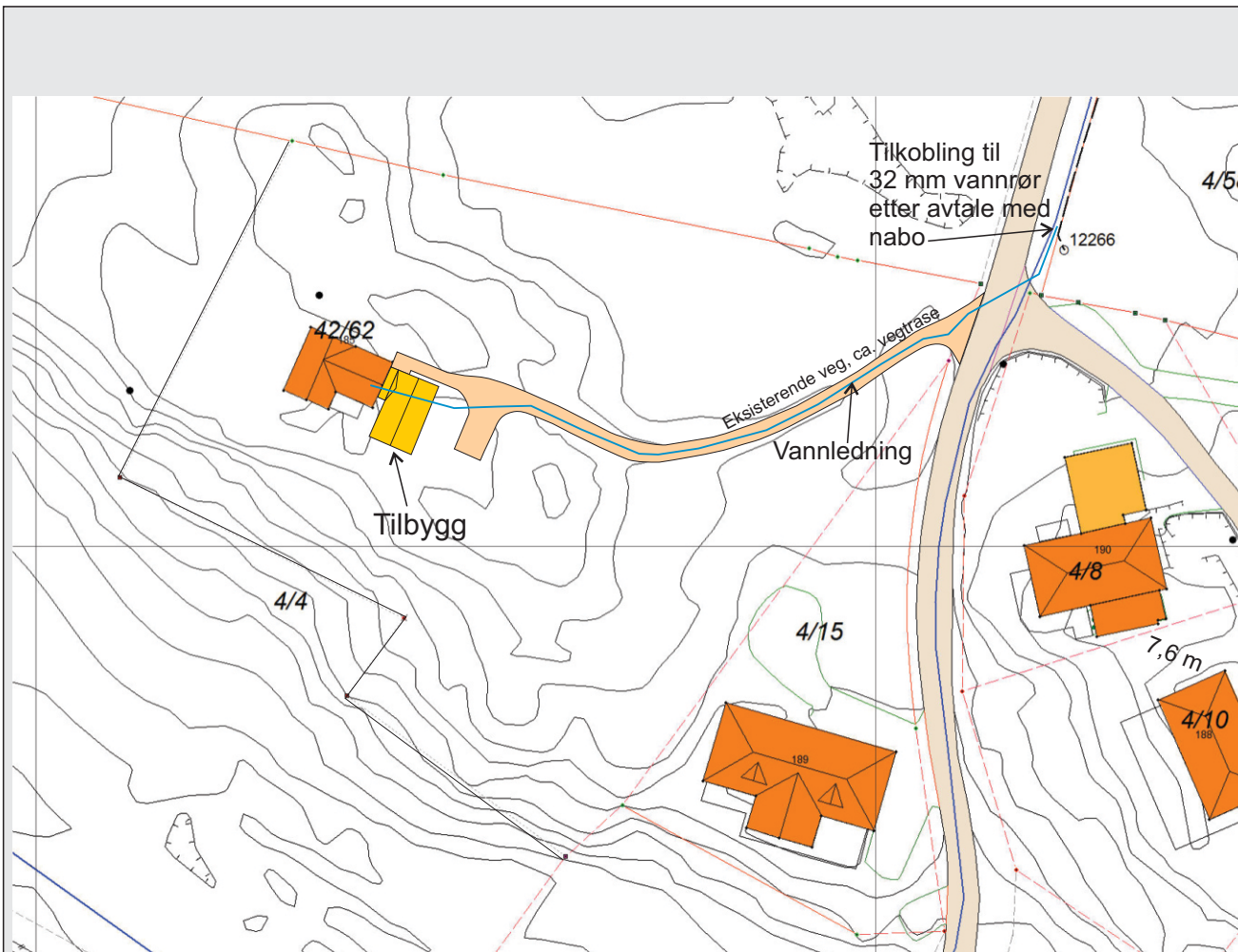
Situasjonsplan vannledningstrase. Trase, vegkryssing og tilkoblingspunkt.
