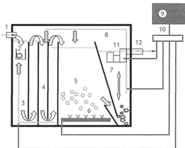
Figur 1. Skisse av rensesanlegget: 1 = innløp, 2 = mekanisk sil, 3 = tilbakepumping av suspendert slam, 4 = anoksisk sone, 5 = aerob sone, 6 = diffusor, 7 = sedimenteringskammer, 8 = returpumping av aerobt slam, 9 = blåsemaskin, 10 = panel for styring av luftinnblåsning, 11 = vannmengderegulering, 12 = utløp.
