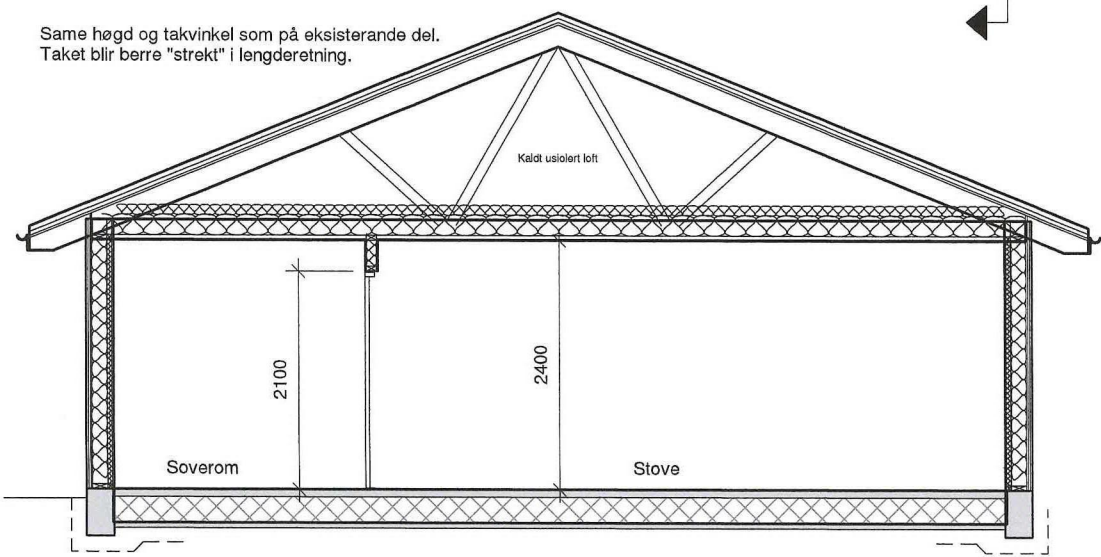
Snitt A-A
