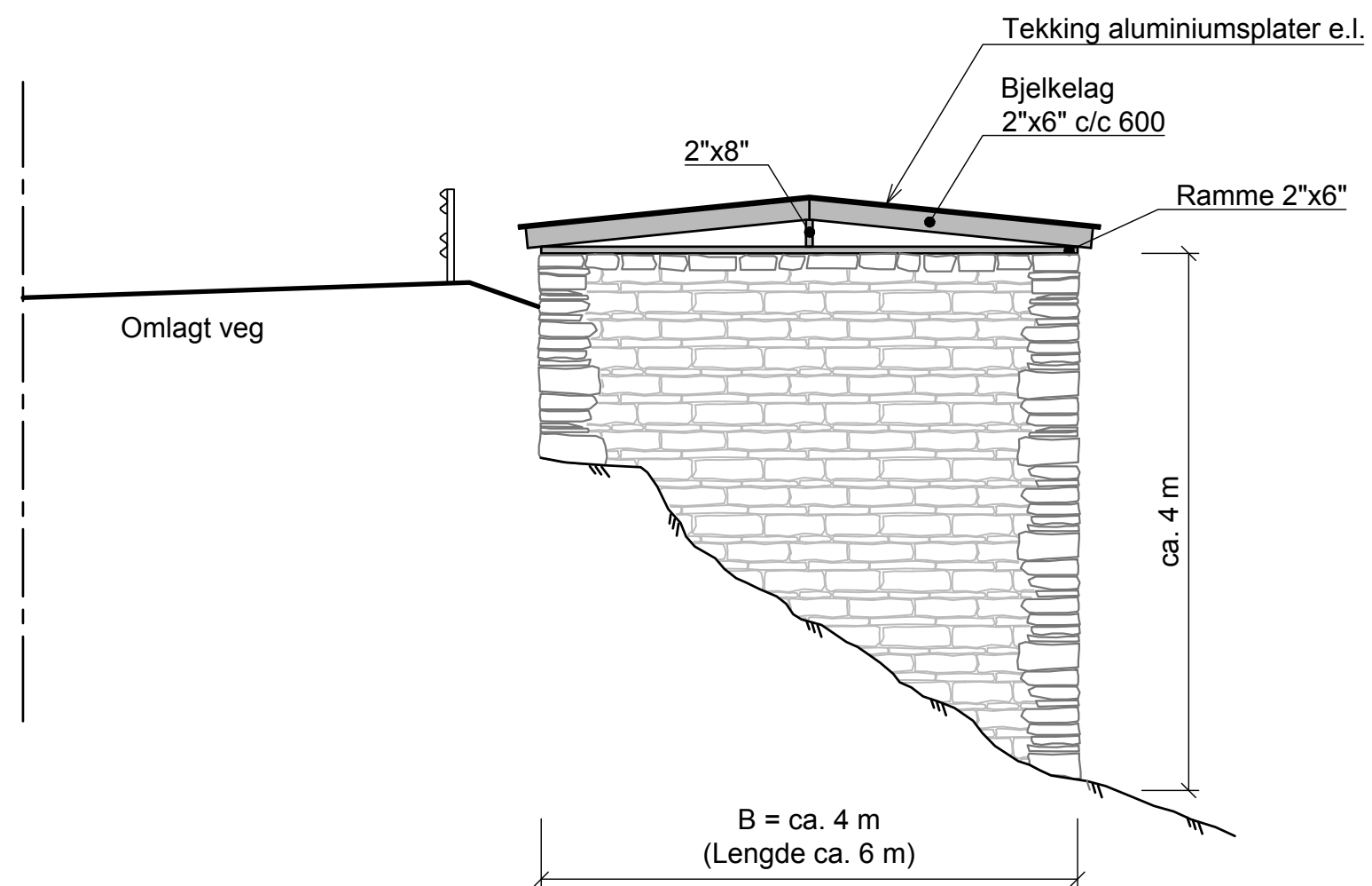
Prinsippskisse sikring mur vedhus
