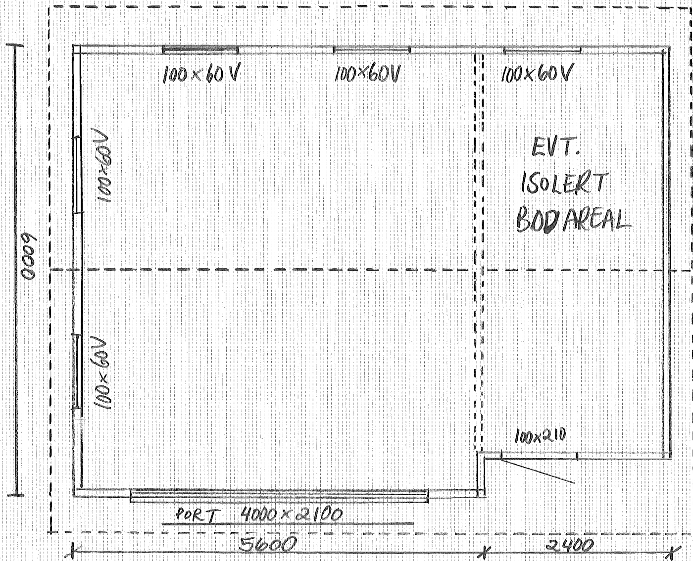
Plantegning mål 1:50
