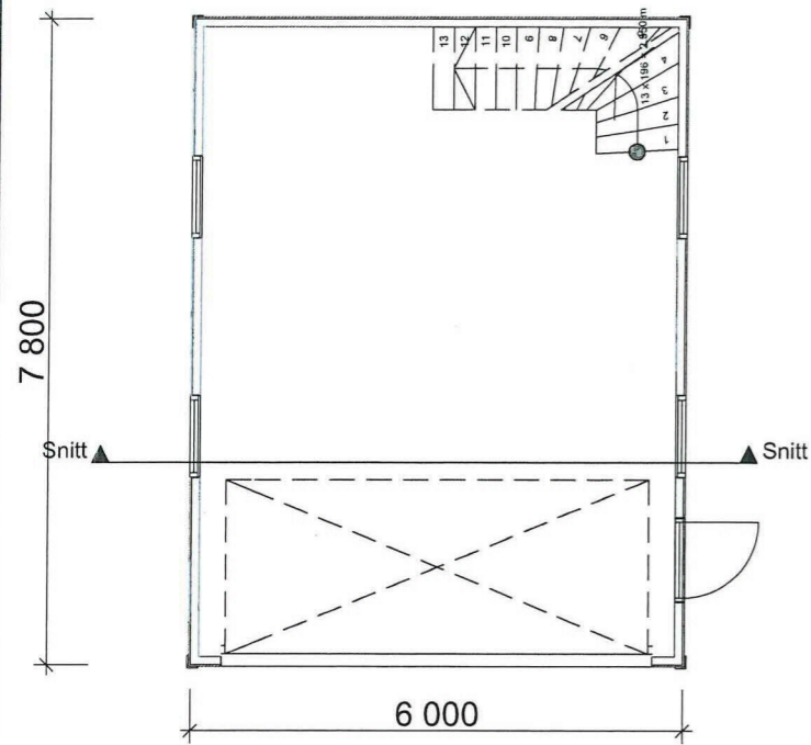
Plan 1 etasje 1:100
