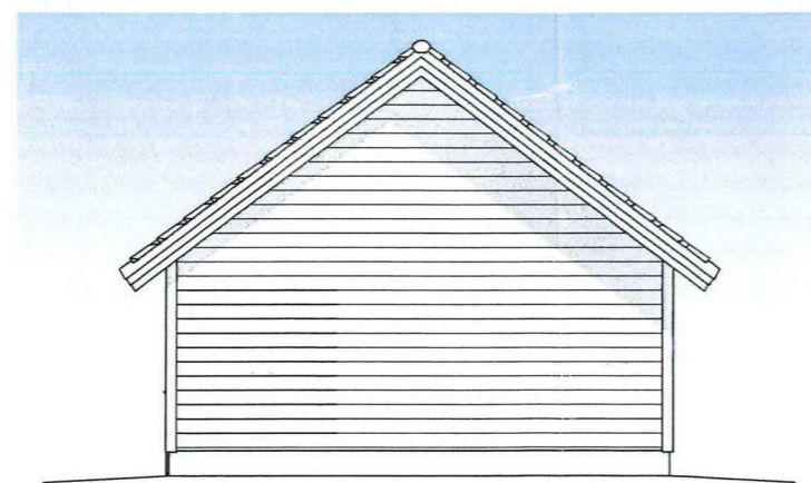
Fasade 2 1:100
