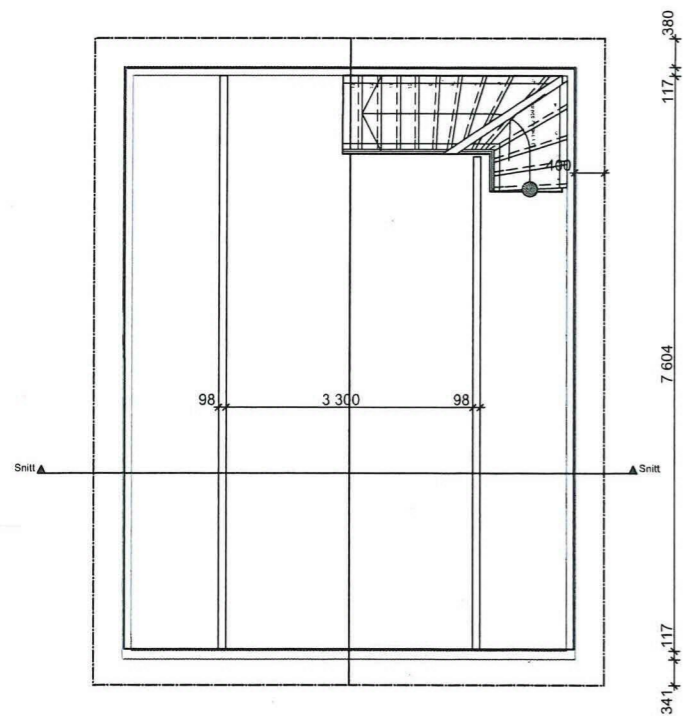
Plan 2 etasje 1:100
