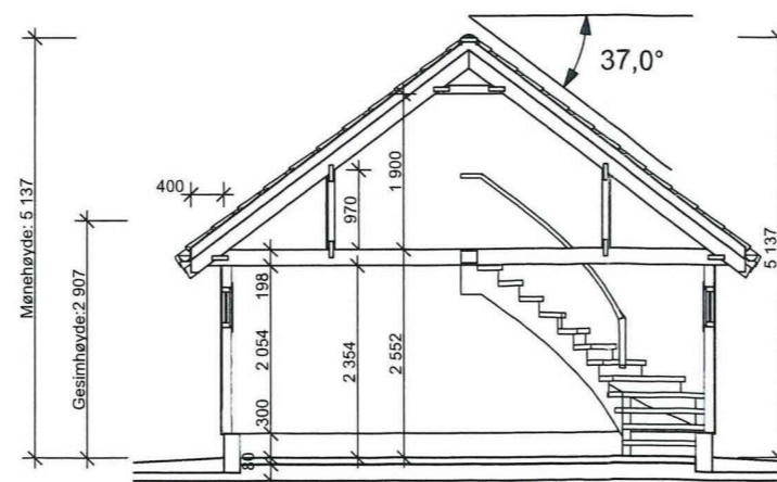
Snitt (1) 1:100
