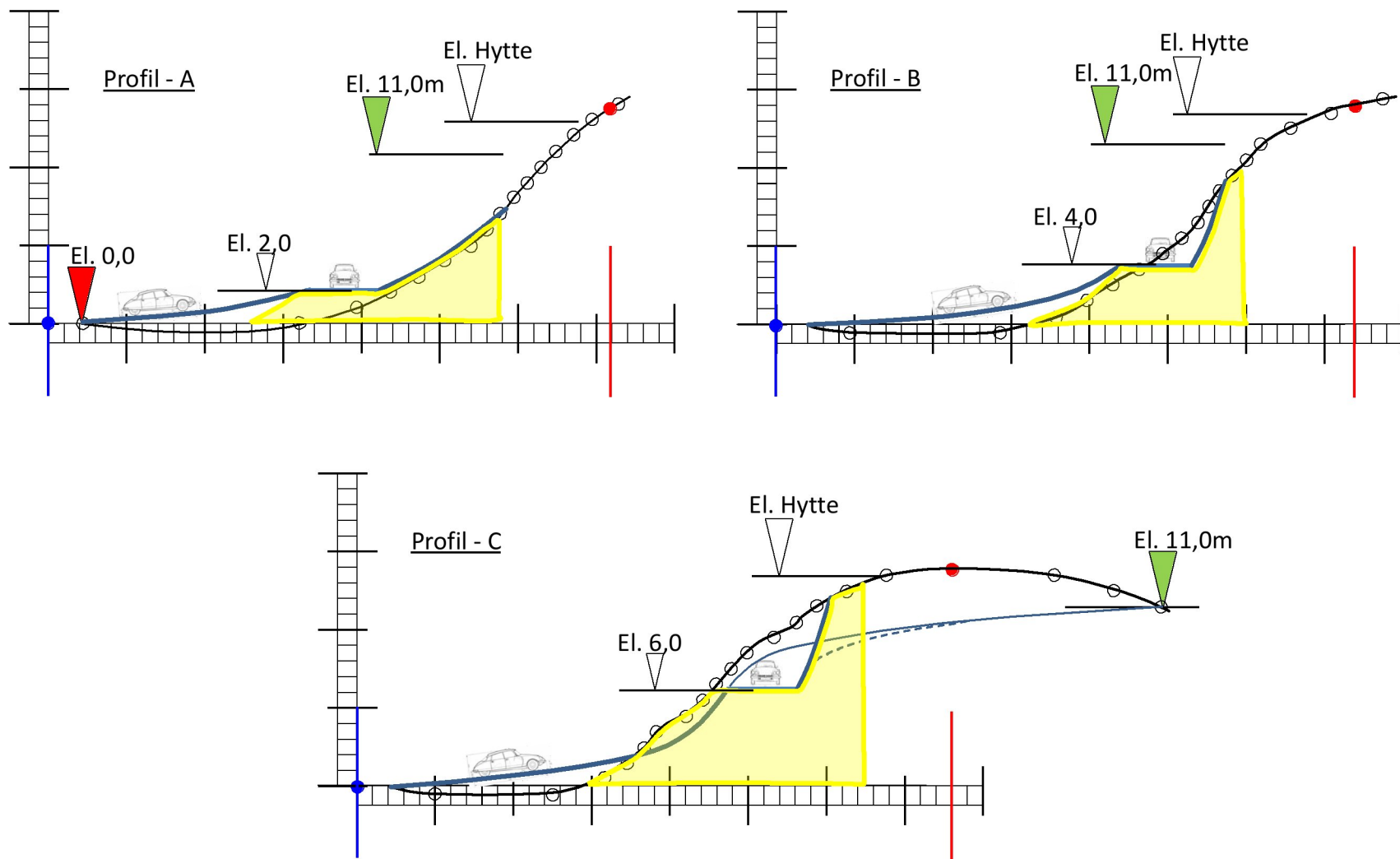
Figur 3 – Vei profil (masser ikke optimalisert)
