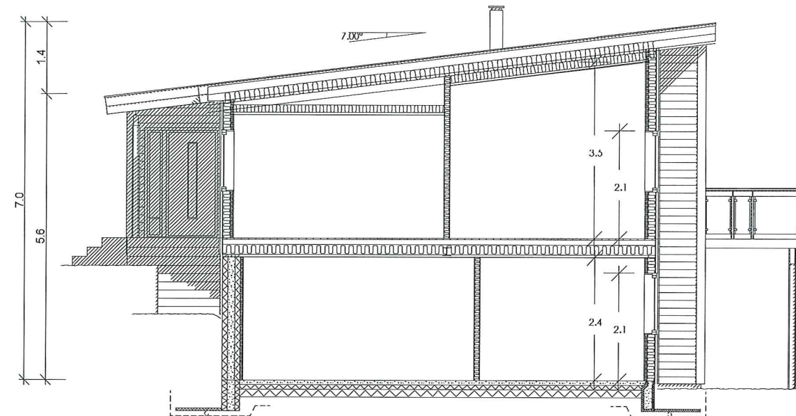
SNITT B-B
