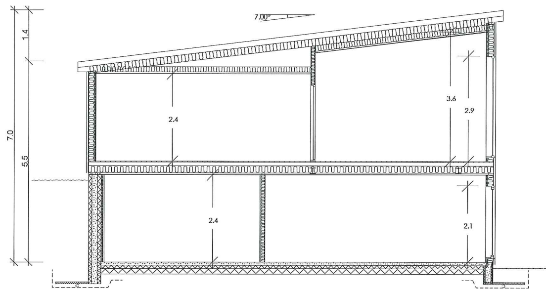
SNITT A-A
