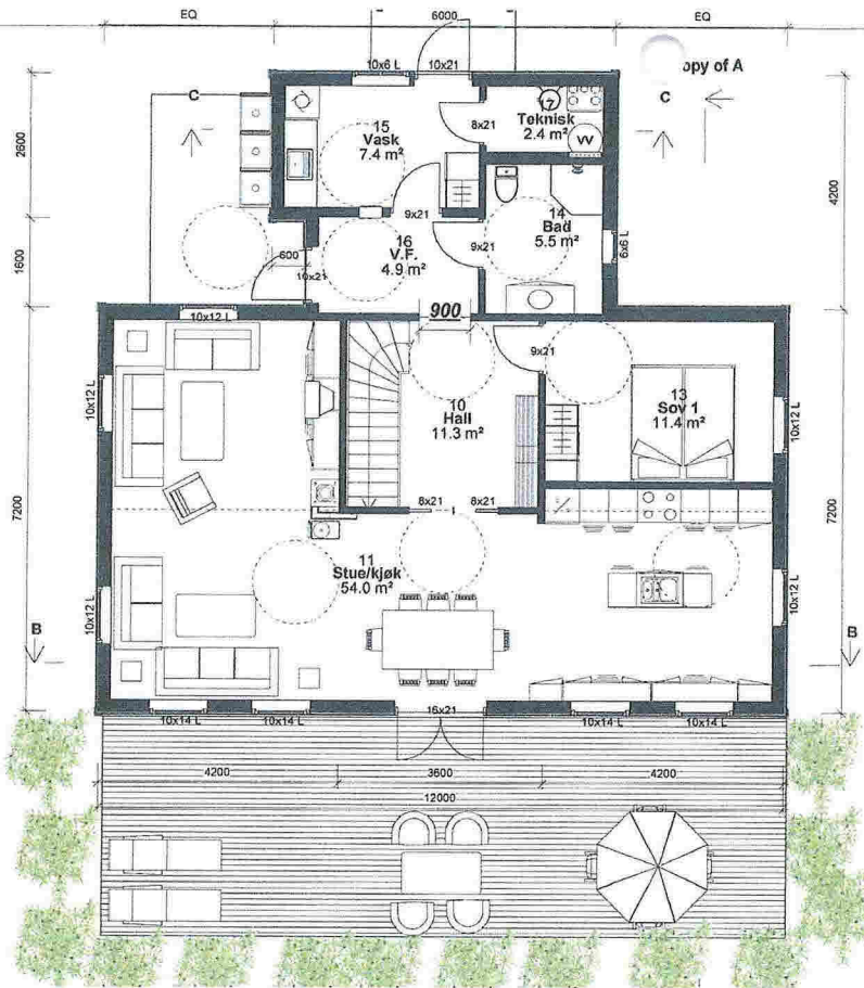
2.0 Hovedetasje 1 : 100
