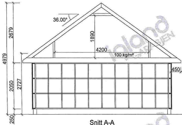
Snitt A-A
