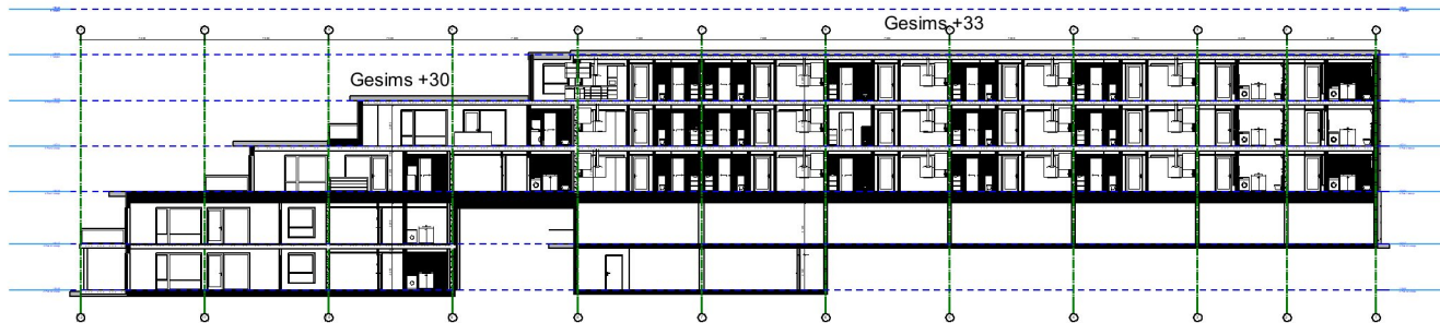
Prinsippsnitt
