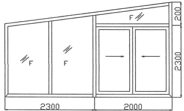
Left Wall
