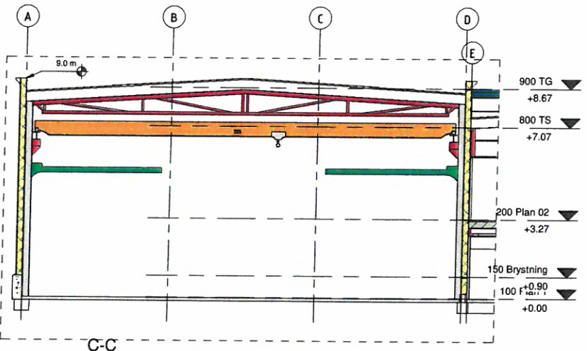
C-C 1 : 100
