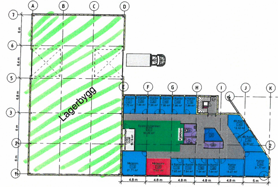
200 Plan 02 1 : 200
