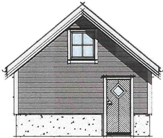
1 Nord 1 : 50
