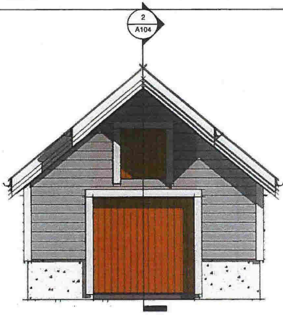
2 Sør 1 : 50
