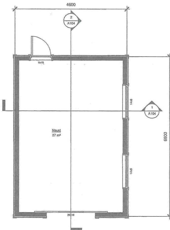
1 Hovedetasje 1 : 50
