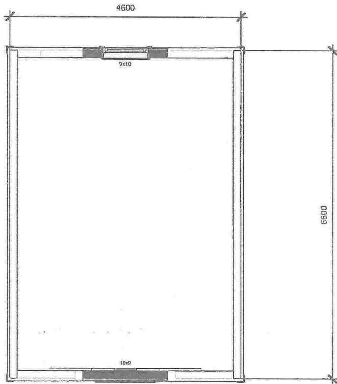
1 Loft 1 : 50
