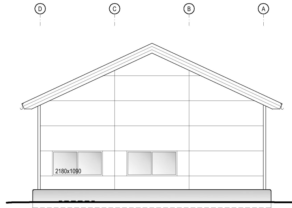
FASADE C
