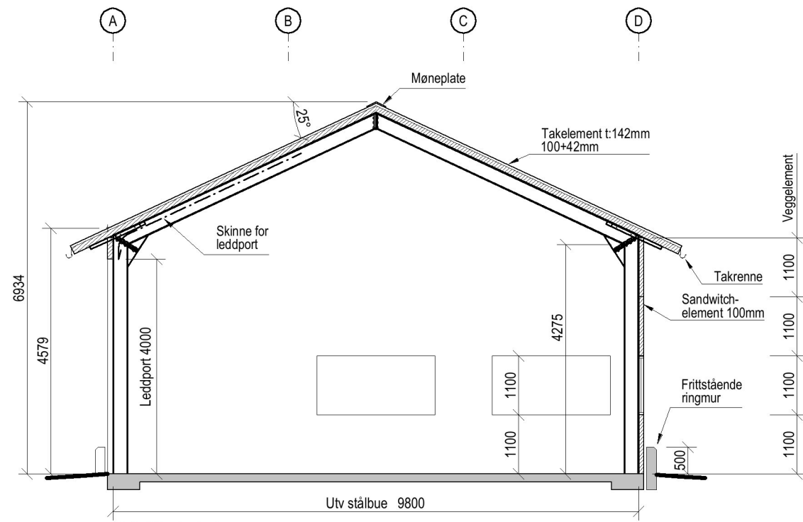
SNITT 1
