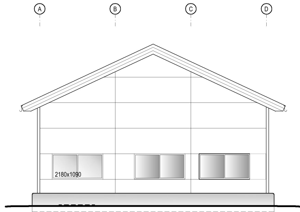
FASADE A
