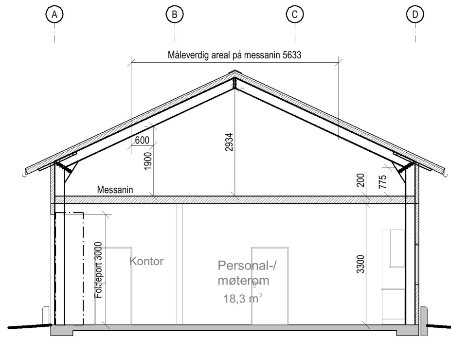
SNITT 2
