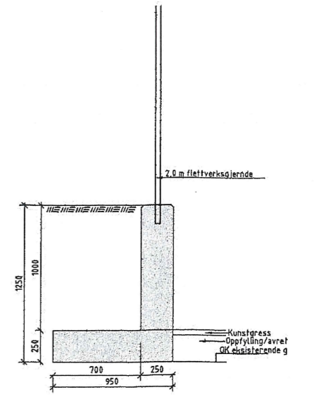
Snitt 2-2 1:20
