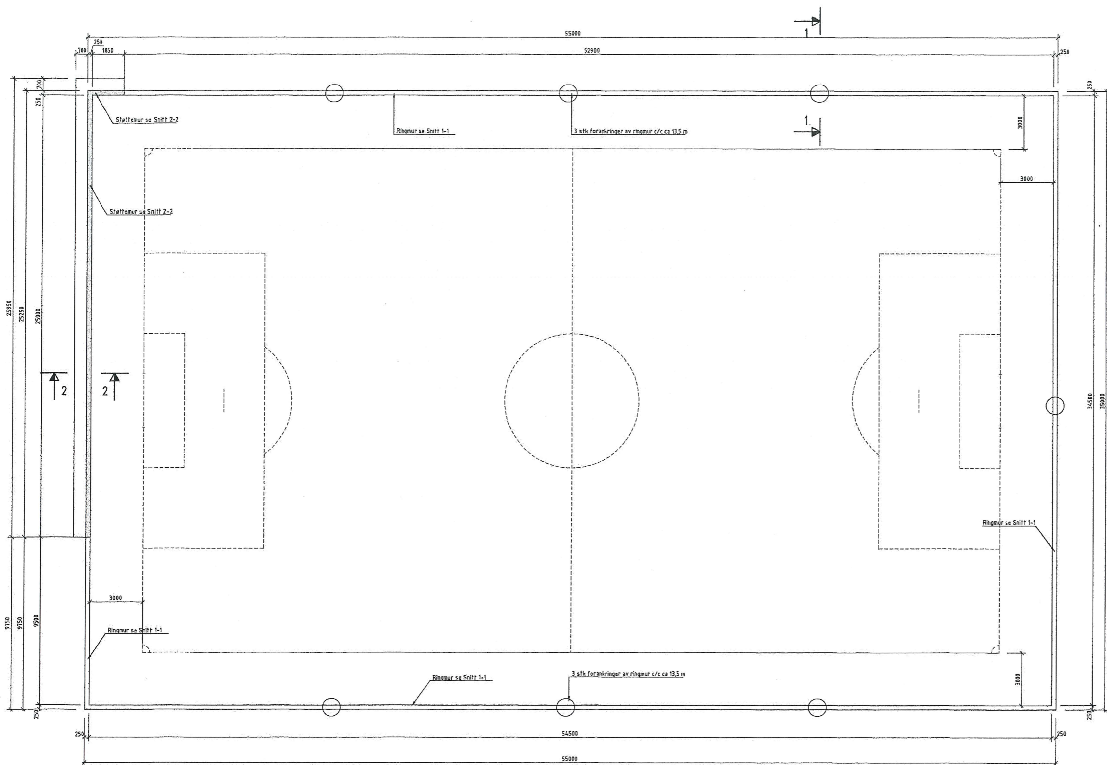
Plan 1:100
