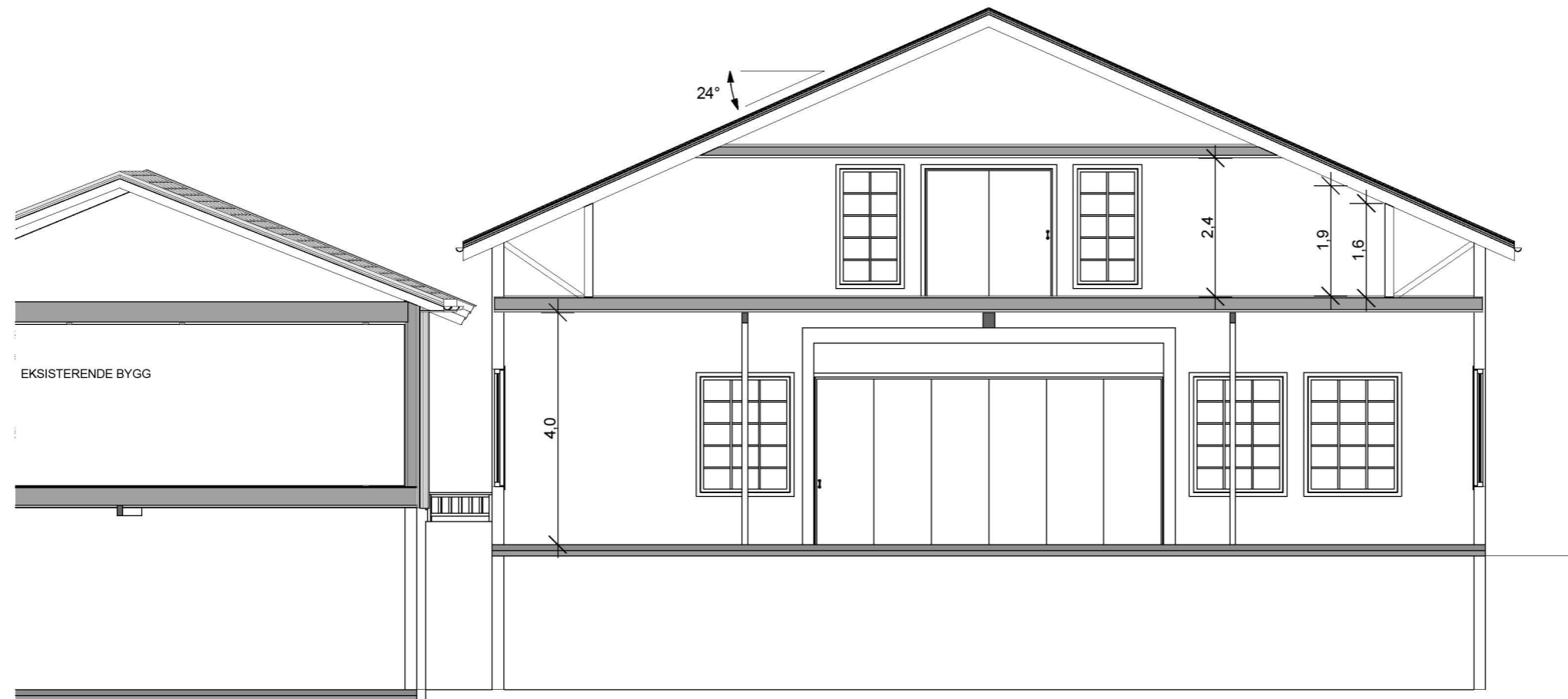
SNITT B-B
