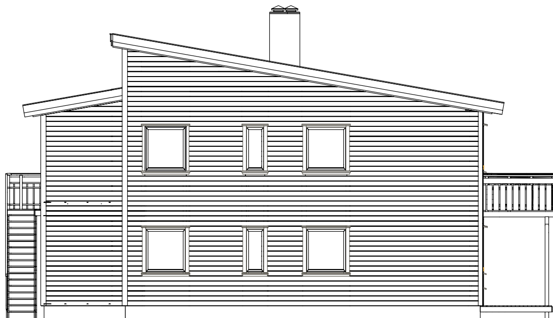
Fasade Nord
