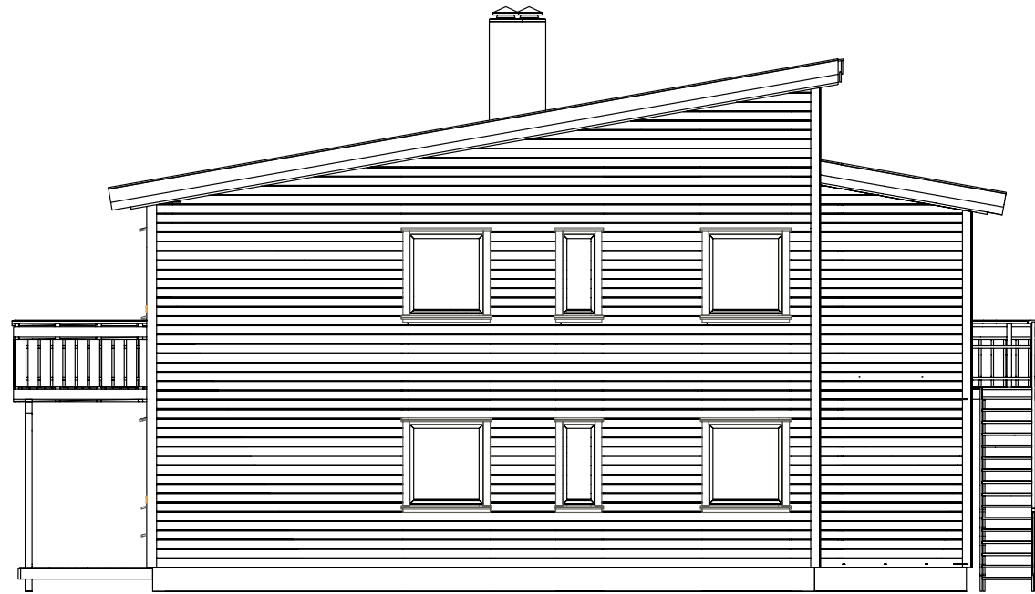
Fasade Sør
