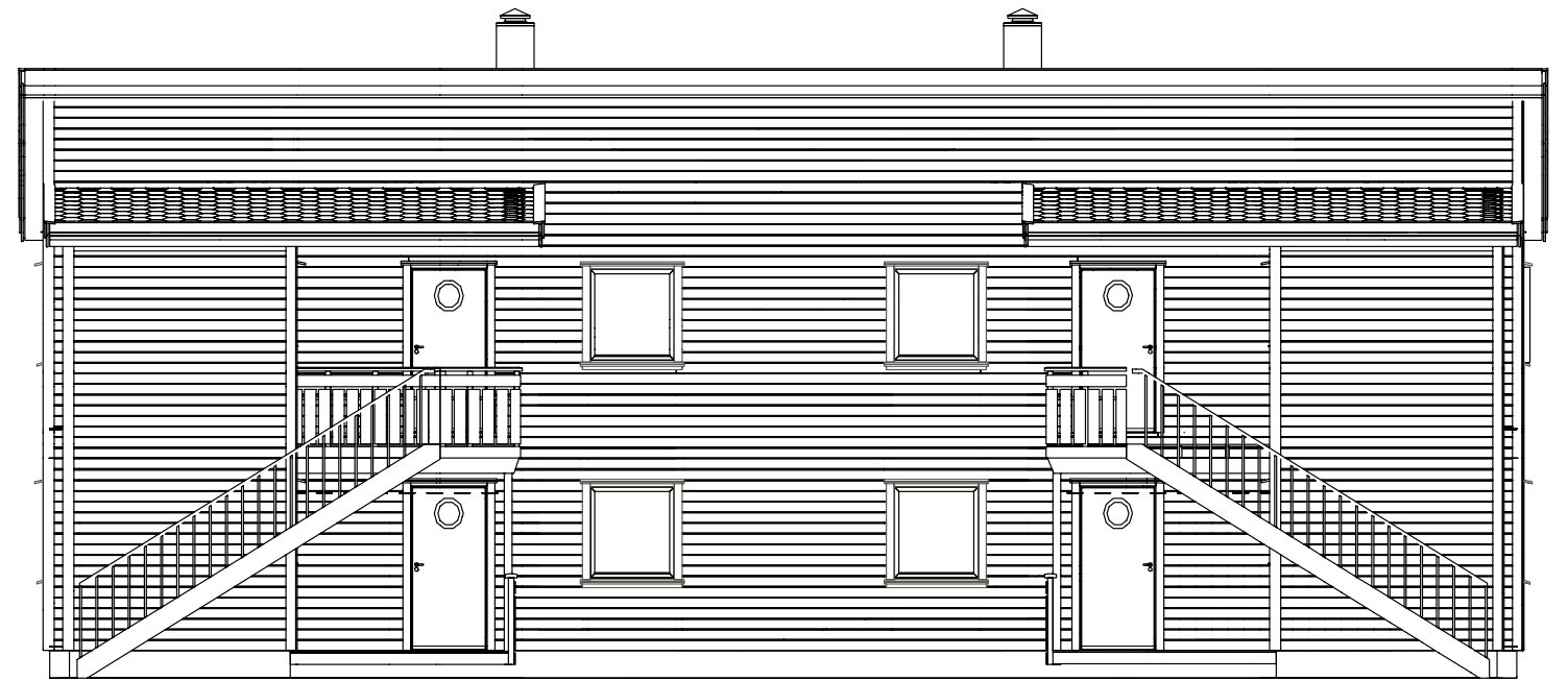
Fasade Øst
