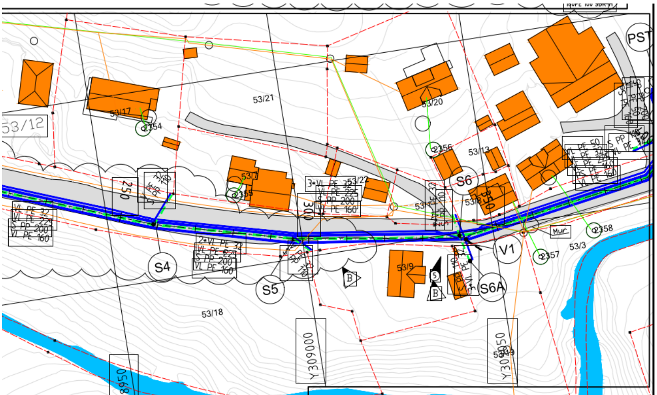
Utklipp 2; utklipp frå arbeidsteikning på aktuell stad.
