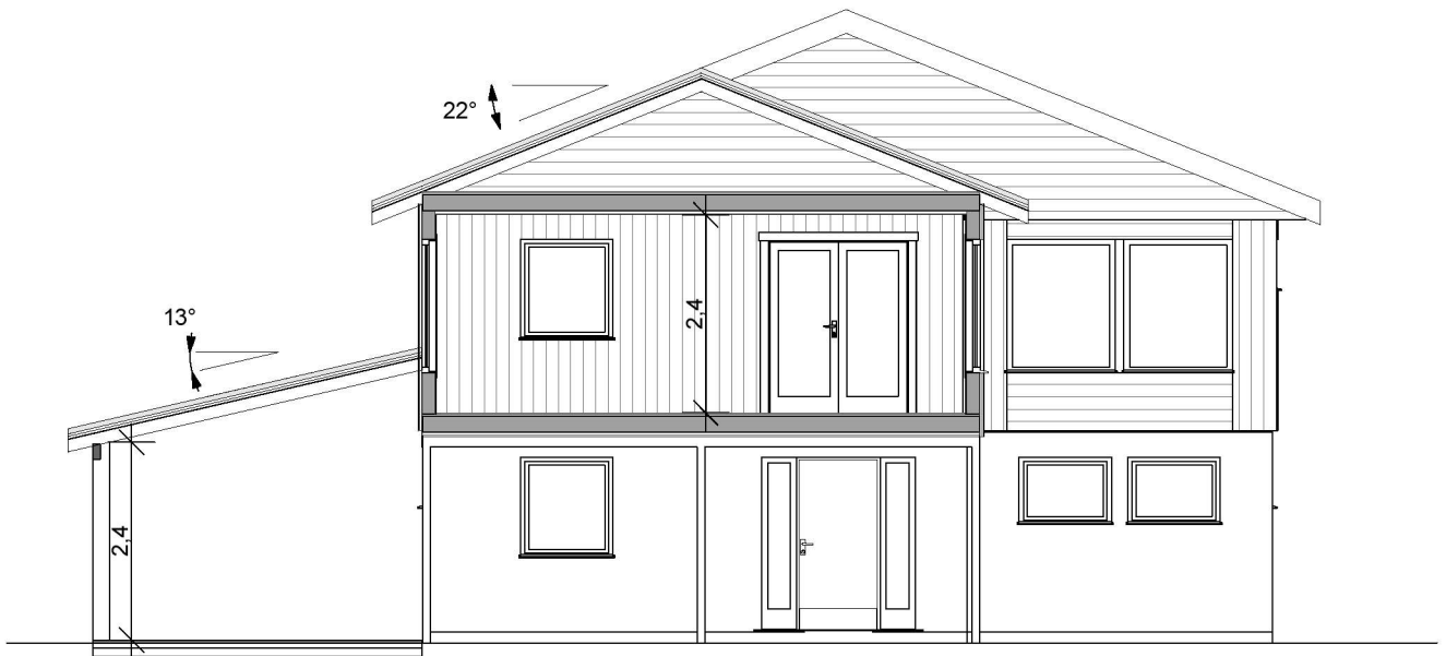
SNITT B-B
