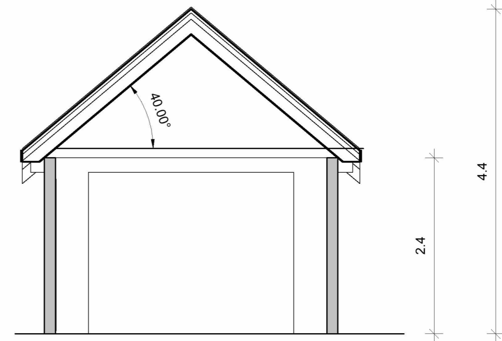
8 Snitt A-A 1 : 50
