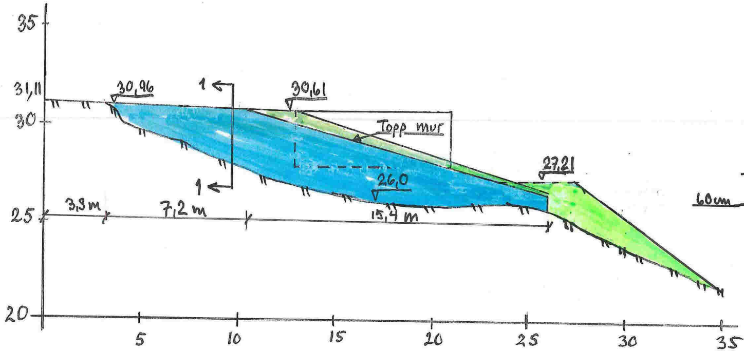
snitt 1-1
