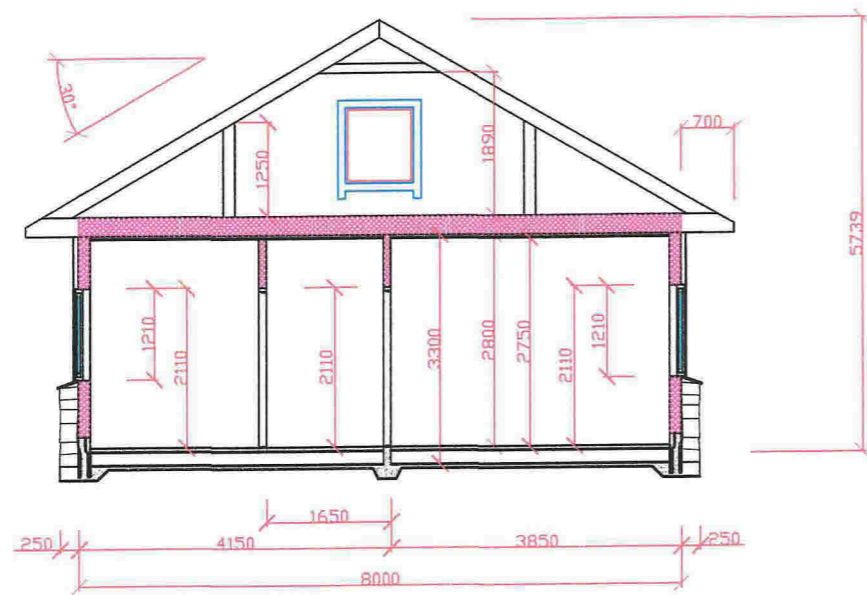
SNITT A-A
