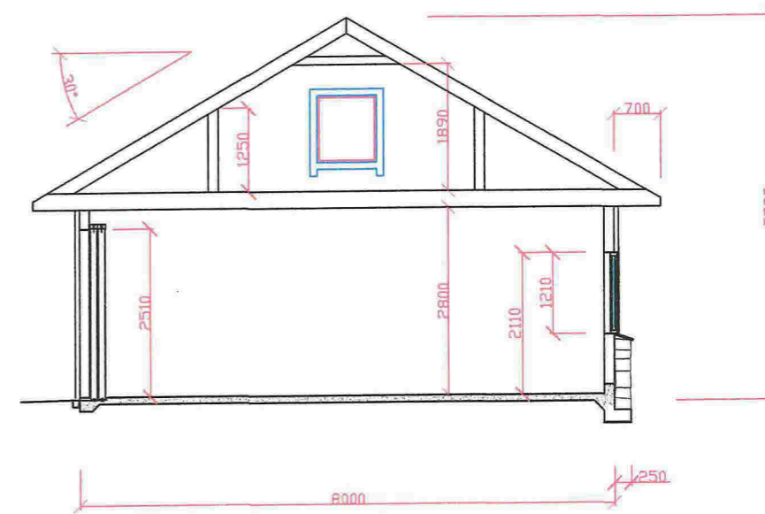
SNITT B-B
