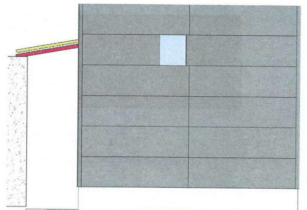
Fasade øst 1:50
