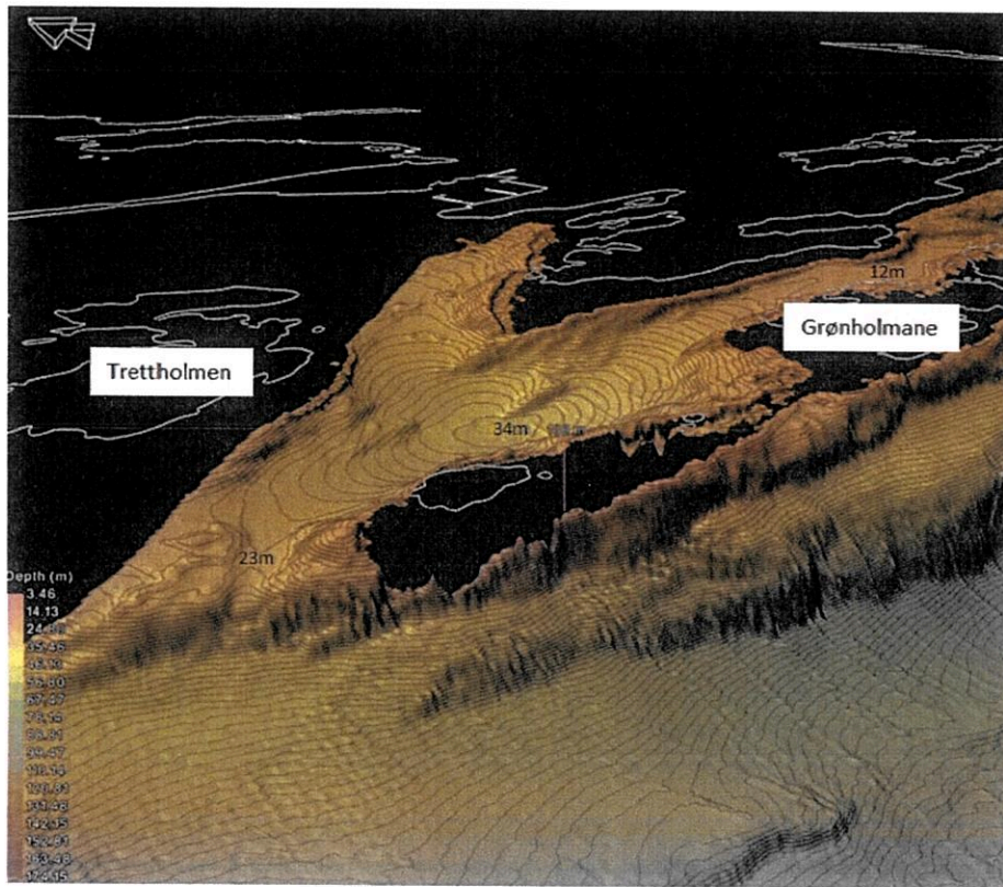
Figur 4.2 MBE dybde data område 1
