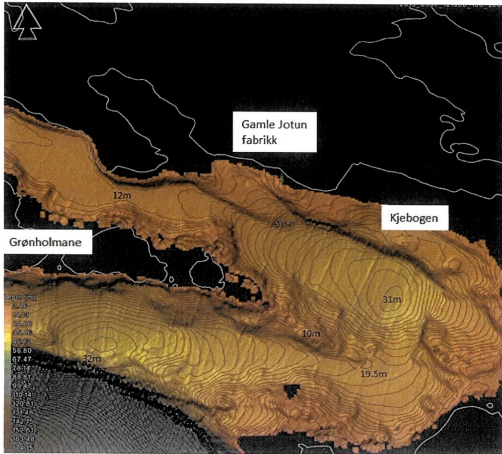
Figur 4.3 MBE dybde data område 1 Kjevogen
