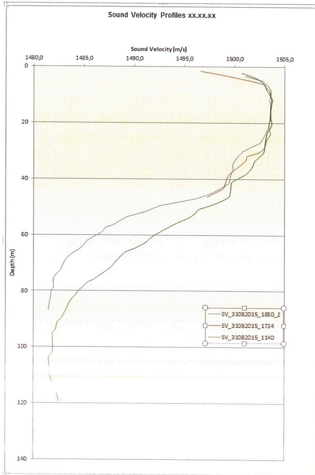
Figur 5.1 Lydhastighetsmålinger logget 31. Aug 2015
