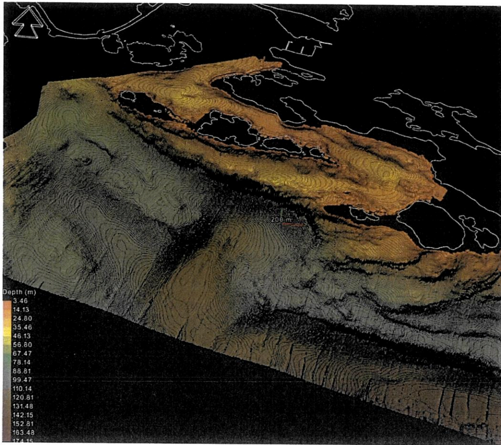
Figur 2.2 DTM of EM3002 data i Kjevogen området sett fra sør
