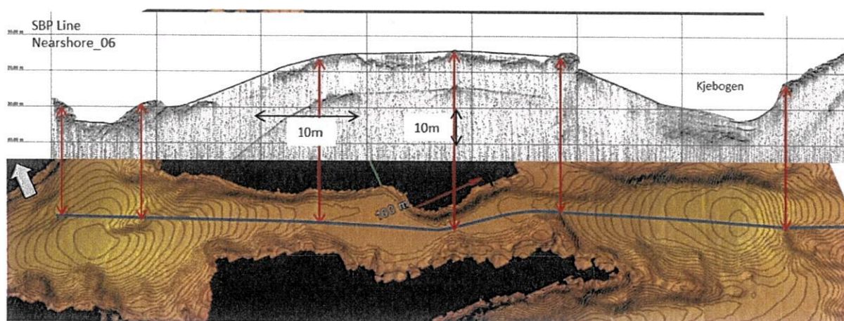
Figur 4.5 SBP og MBE område 1 (røde piler – antatt bart berg)
