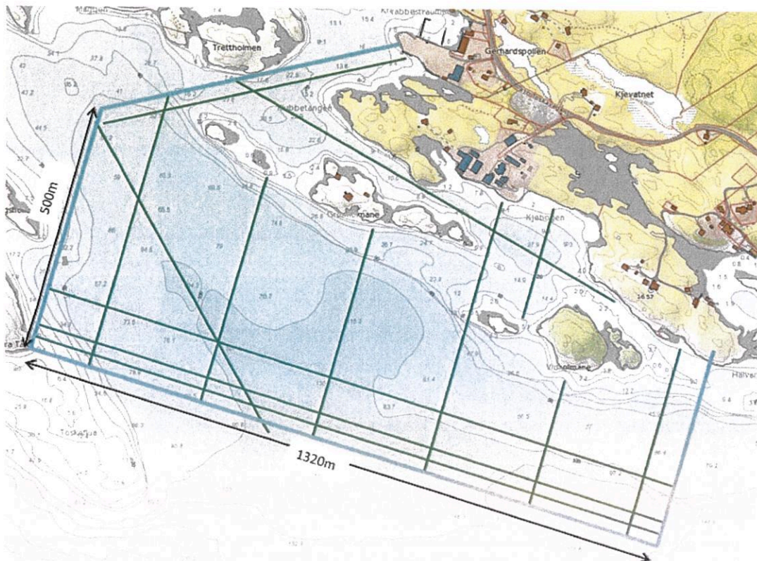
Figur 4.1 Survey området SBP linjer (grønn)
