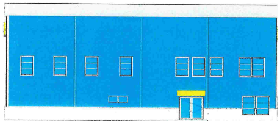
1 Sør-øst 1 : 100
